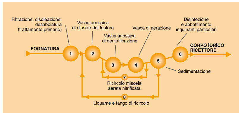
Schema di un impianto di depurazione
