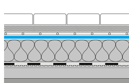
COPERTURA PRATICABILE
