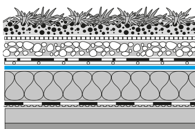
GIARDINO PENSILE
